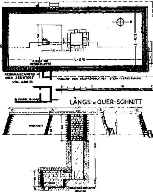
تخطيط أرضى ومقطع رأسى لمقبرة من الأسرة الرابعة «رسم هـ. يونكر»
